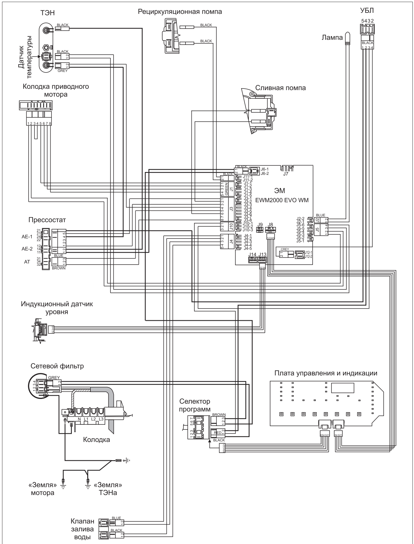
Рис. 4. Монтажная схема СМ «Electrolux EWF1234» с модулем EWM2000 EVO
