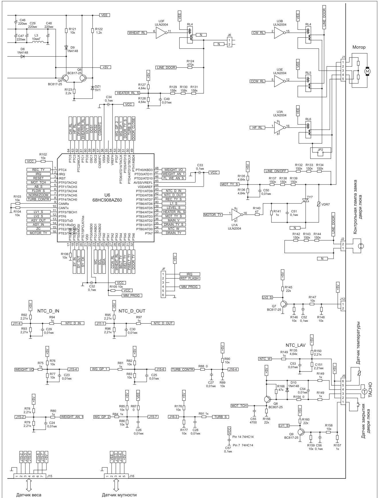
Рис. 2. Принципиальная электрическая схема ЭМ EWM2000 EVO (2/2)
