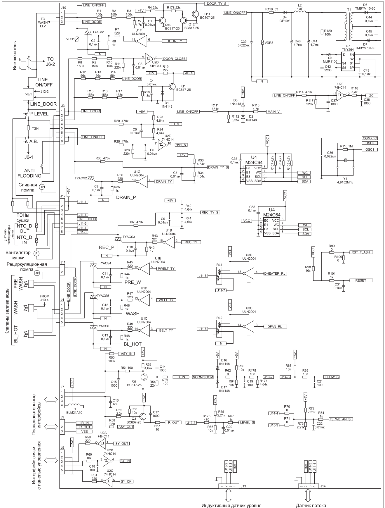
Рис. 2. Принципиальная электрическая схема ЭМ EWM2000 EVO (1/2)
